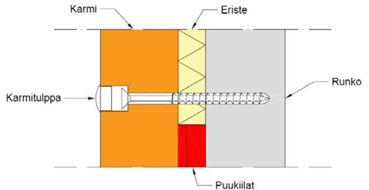
Kuva 3. Ruuvikiinnitys, pystyleikkauskuva
