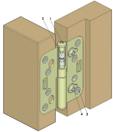
Kuva 1. Saranan säätö
